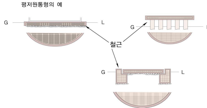
그림 2.2.2.3 저장탱크의 수평기초면
