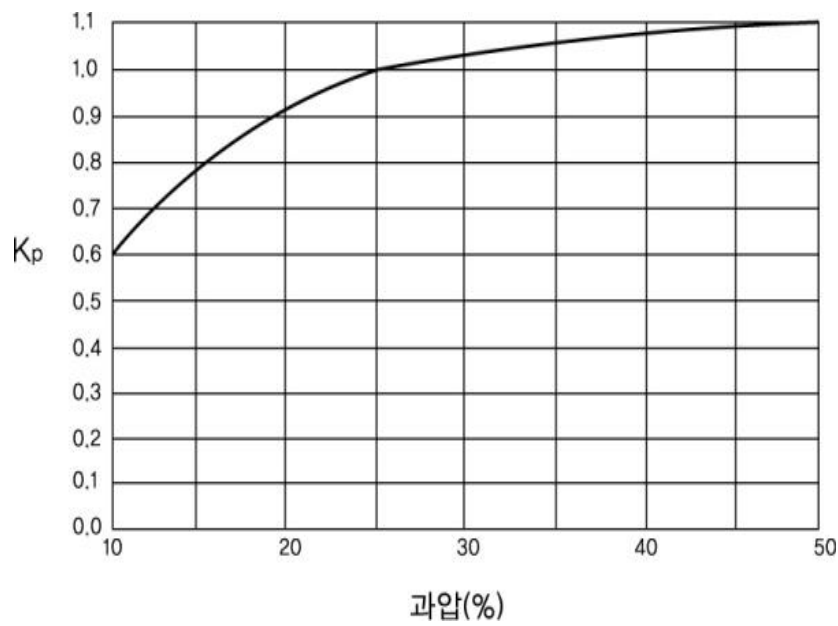
그림 2.7.1.4.2③ 과압보정계수
