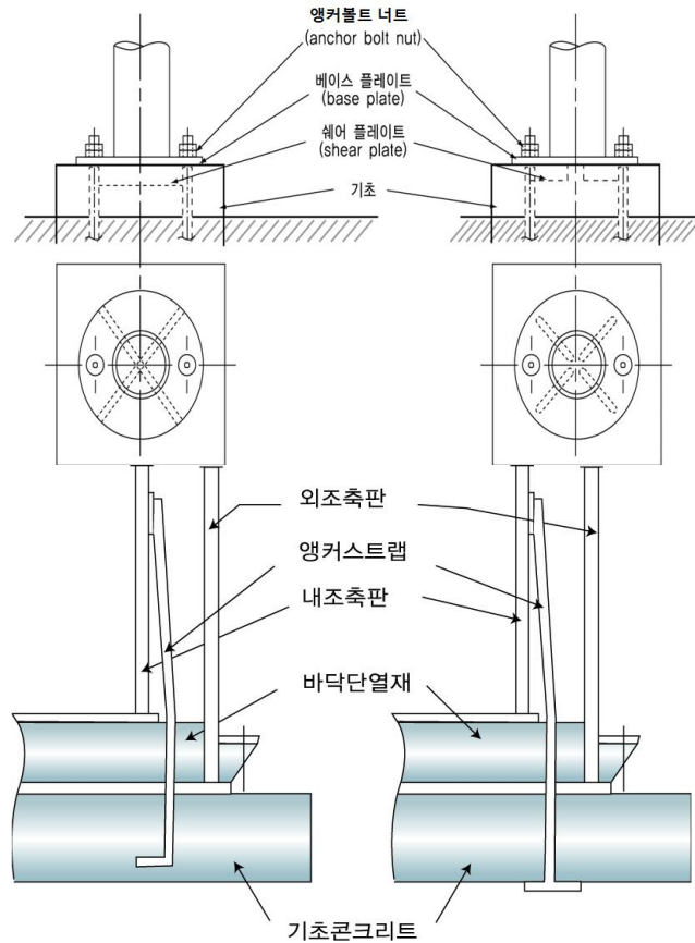
그림 2.2.3.7 평저형 저장탱크의 앵커스트랩 설치방법
