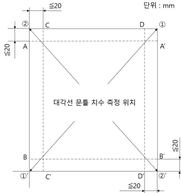
그림 3.2 방호문의 치수측정 위치
