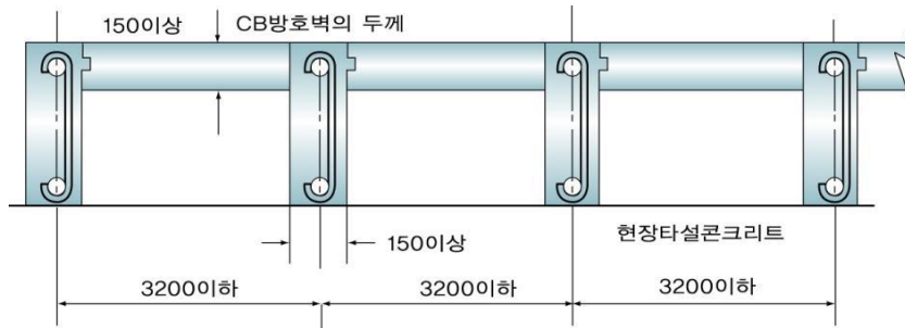
그림 2.7.2.2.2 보조벽의 배치
