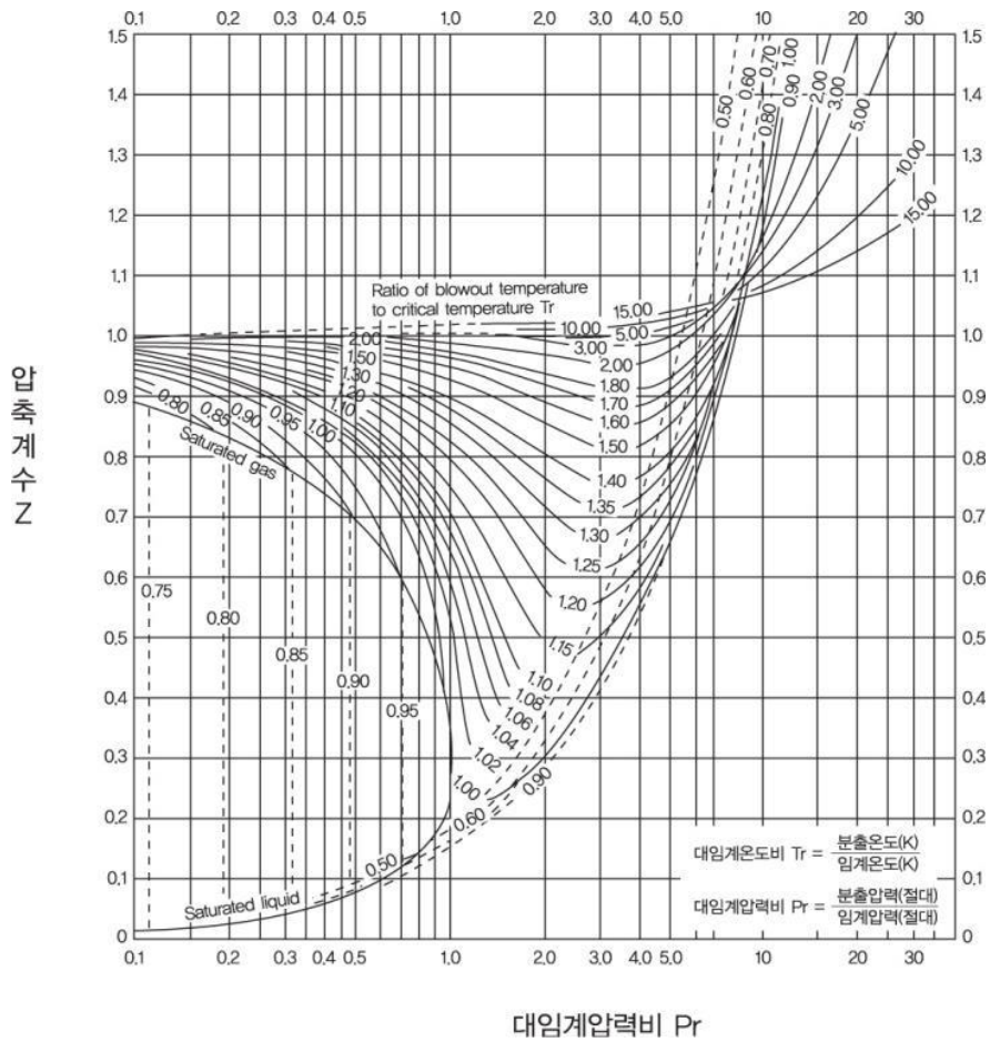
그림 2.6.1.4④ 압축계수
