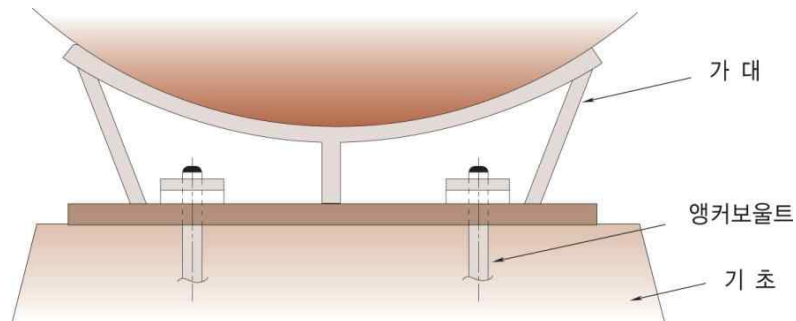
그림 2.2.3.4 앵커보울트의 고정방법
