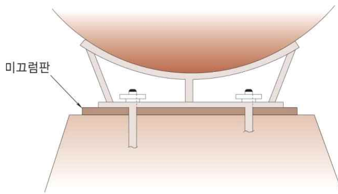
그림 2.2.3.5.3 미끄럼판의 설치방법
