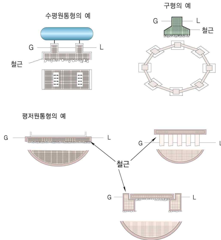
그림 2.2.2.3 저장탱크의 수평기초면
