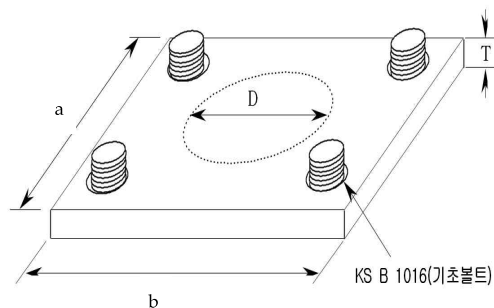
그림 2.4.4.2.1(6-4-2) 강관제 보호대의 받침대 설치 방법
