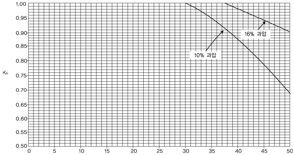
그림 2.6.1.4② 밸런스 벨로즈형 안전밸브 배압보정계
