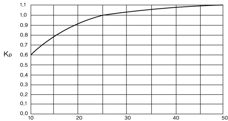
그림 2.6.1.4⑧ 과압보정계수
