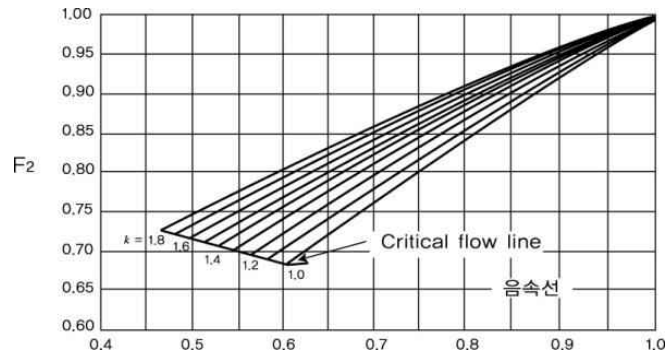
그림 2.6.1.4⑤ 아음속계수
