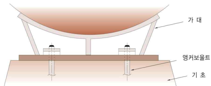
그림 2.2.3.4 앵커볼트의 고정방법
