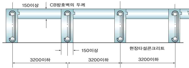
그림 2.7.2.2.2 보조벽의 배치
