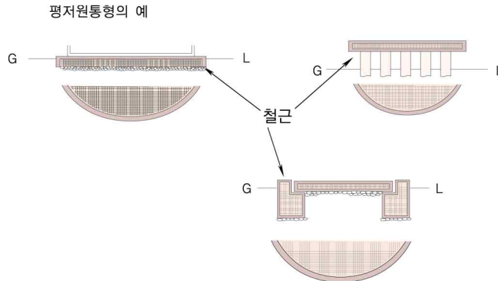
그림 2.2.2.3 저장탱크의 수평기초면
