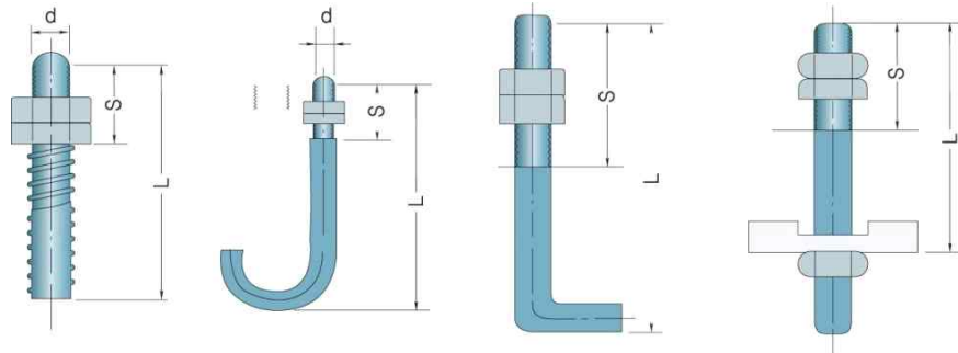
그림 2.2.3.3 앵커볼트의 치수표시
