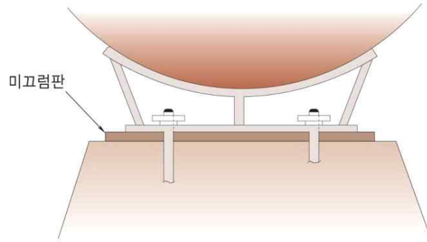
그림 2.2.3.5 미끄럼판의 설치방법
