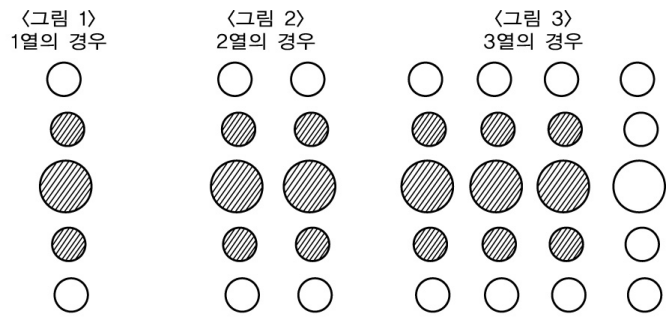
주) 사선 친 부분의 저장탱크가 대상표면적이 됨. 그림 2.7.9.1.4 온도상승방지설비 능력 산정 기준
