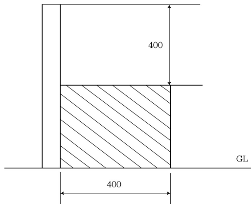
그림 2.7.2.2.3 보조벽의 높이
