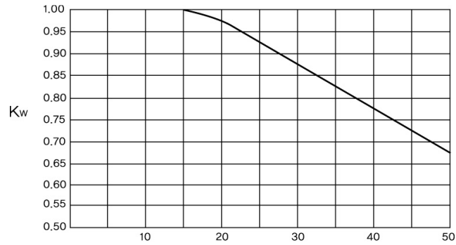
그림 2.6.1.4⑥ 벨런스 벨로우즈형 안전밸브 배압보정계수
