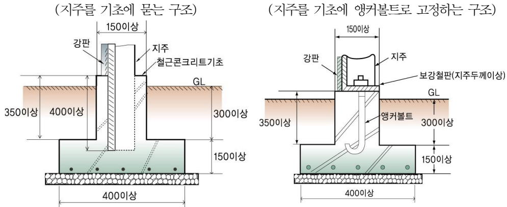
그림 2.7.2.3.6 강관제 방호벽의 고정방법 보기
