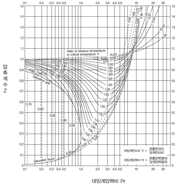
그림 2.6.1.4④ 압축계수
