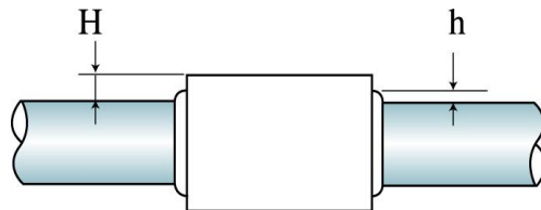
그림 2.5.4.1.4③ 비드높이(h) 및 이음관의 높이(H)
