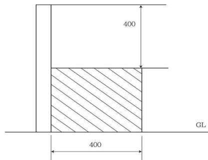
그림 2.7.2.2.4 보조벽의 높이
