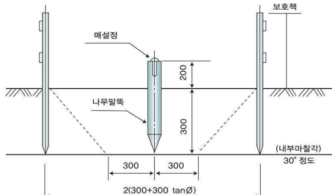
그림 3.1.2.1.1(2) 임시 벤치마크의 설정 예시
