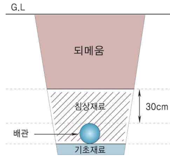
그림 2.5.7.2.5 도매움 구조
