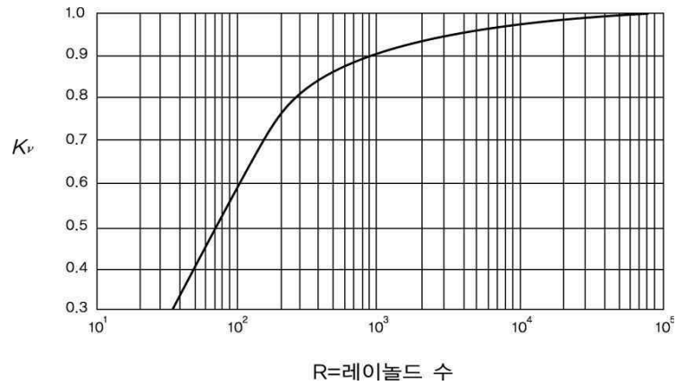
R=레이놀드 수 그림 2.6.1.4(2)⑦ 점도로 인한 용량보정계수
