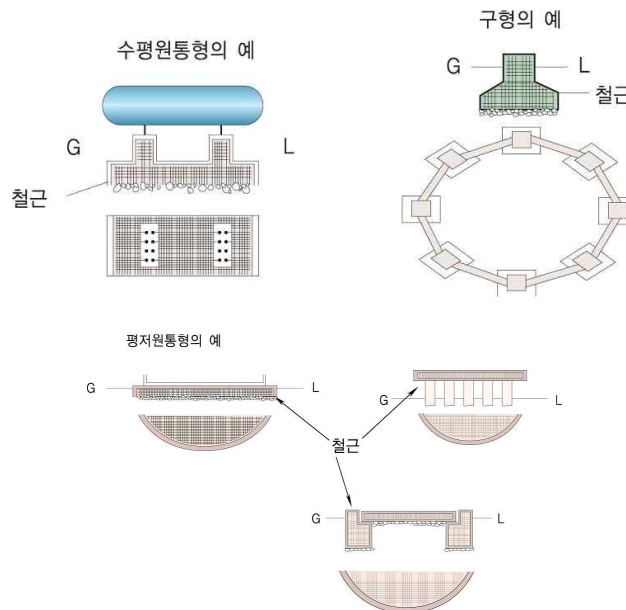
그림 2.2.2.4 저장탱크의 수평기초면
