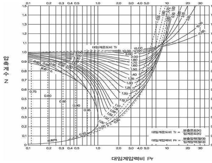
그림 2.6.1.4(2)④ 압축계수
