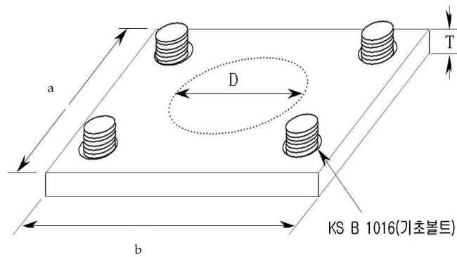
그림 2.3.3.6.5 강관제 보호대의 받침대 설치 방법 <개정 19.8.14>
