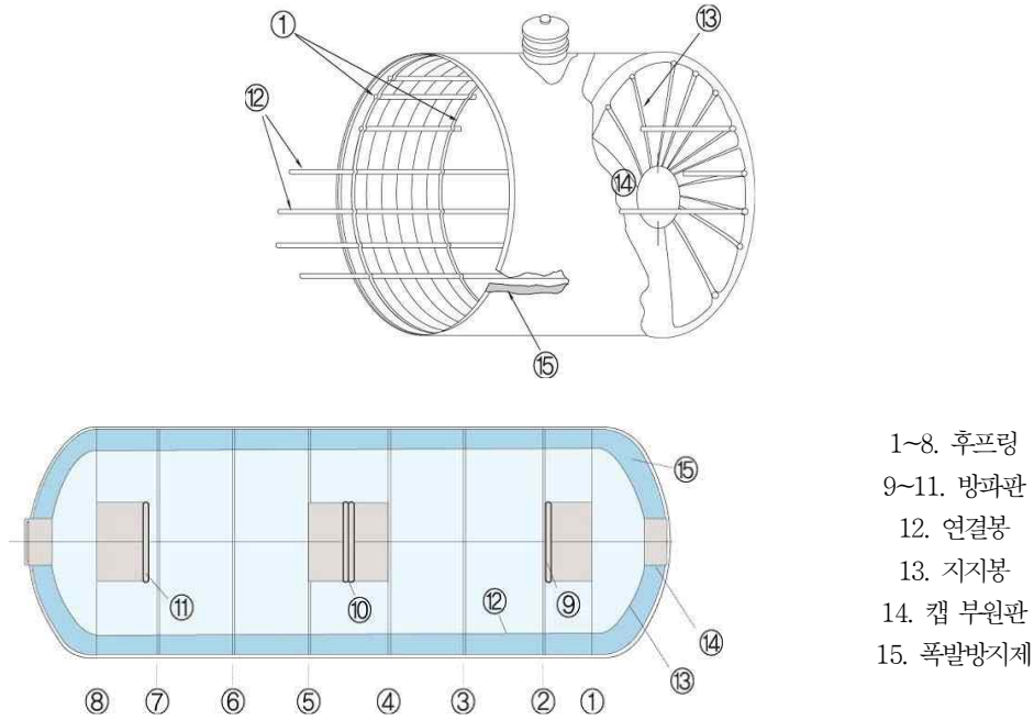
그림 2.3.3.5.1② 폭발방지장치 전체조립도
