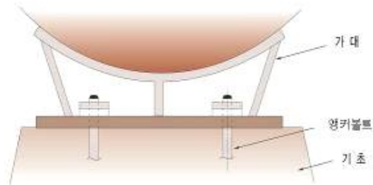
그림 2.2.3.4 앵커볼트의 고정방법
