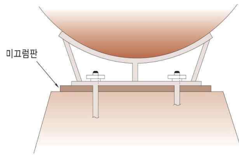
그림 2.2.3.5 미끄럼판의 설치방법
