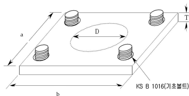
그림 23323(6-4-2) 강관제 보호대의 받침대 설치 방법 &lt;개정 19.8.14&gt;
