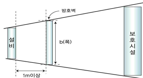
그림 2.1.1.3② 방호벽 설치 예(평면도)
