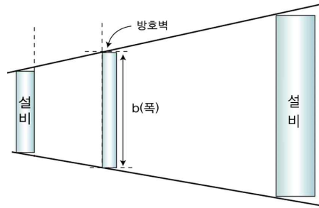
그림 2.7.2.1.3② 방호벽 설치 예(평면도)
