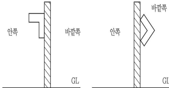
그림 2.7.2.4.2 강관제 방호벽의 앵글강 보강
