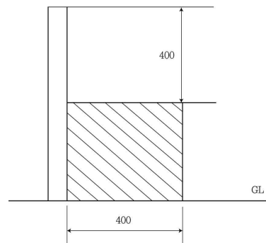
그림 2.7.2.3.3 보조벽의 높이
