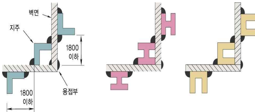
그림 2.7.2.4.4 지주의 설치방법
