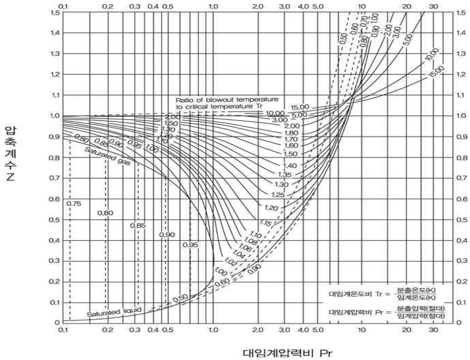
그림 2.6.1.4④ 압축계수
