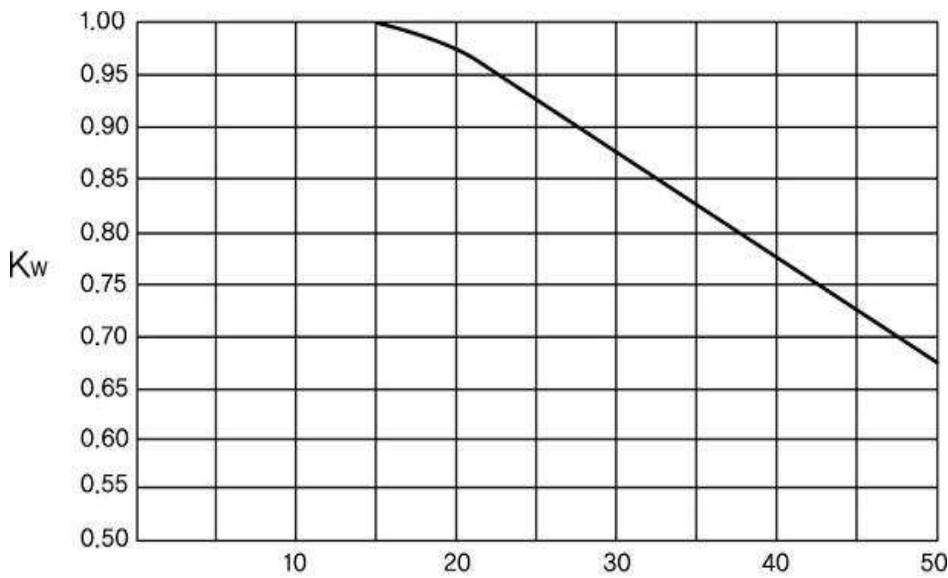
그림 2.6.1.4⑤ 아음속계수
