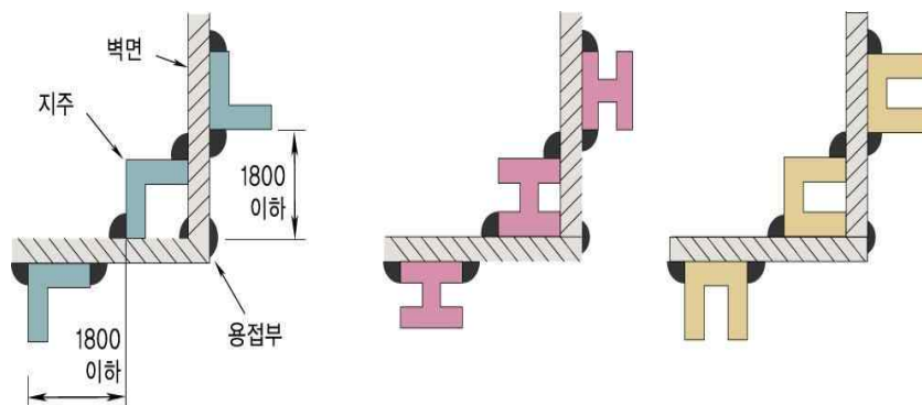
그림 2.7.2.4.4 지주의 설치방법
