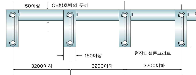
그림 2.7.2.3.2 보조벽의 배치
