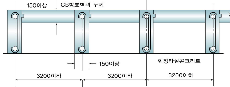
그림 2.7.2.2.2 보조벽의 배치
