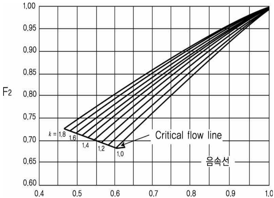
그림 2.6.1.4④ 압축계수
