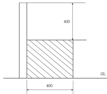
그림 2.7.2.3.3 보조벽의 높이
