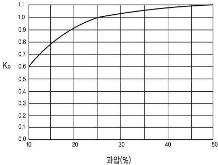
그림 2.6.1.4⑧ 과압보정계수
