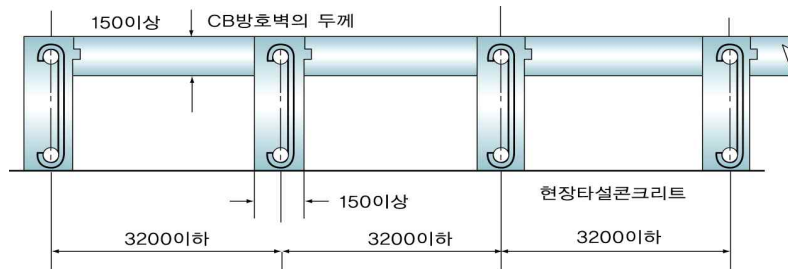
그림 2.7.2.3.2 보조벽의 배치
