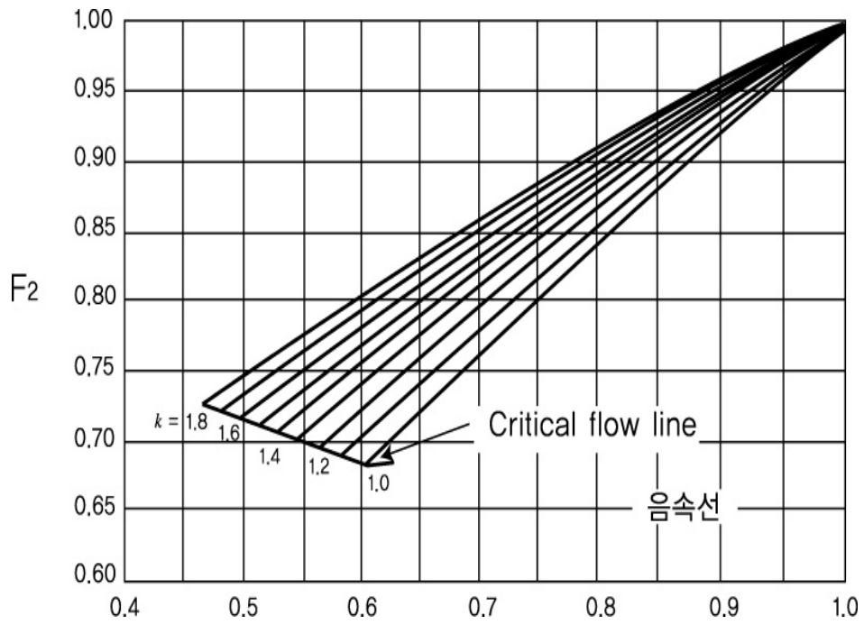
그림 2.6.1.4⑤ 아음속계수
