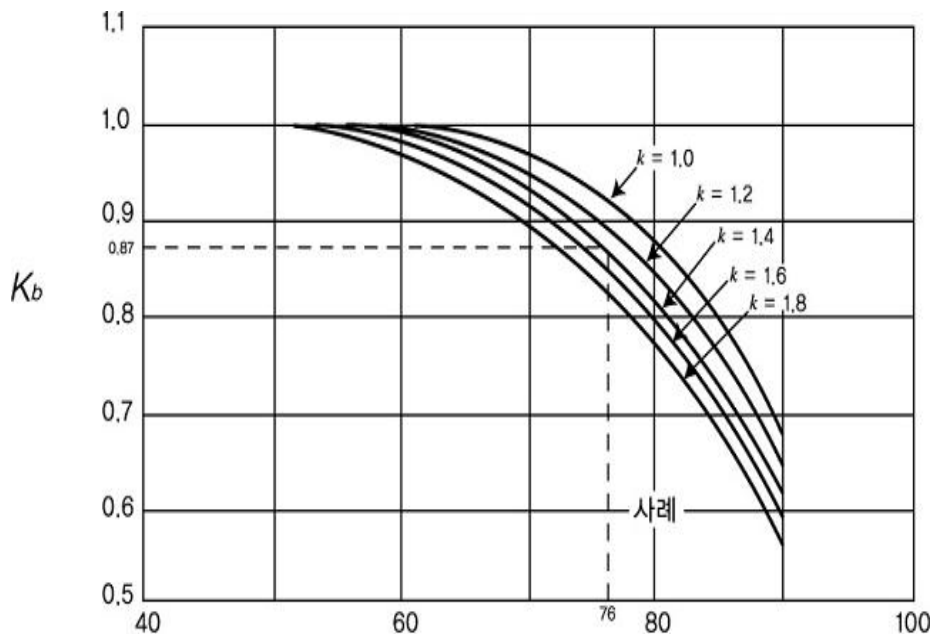
그림 2.6.1.4② 밸런스 벨로우즈형 안전밸브 배압보정계수
