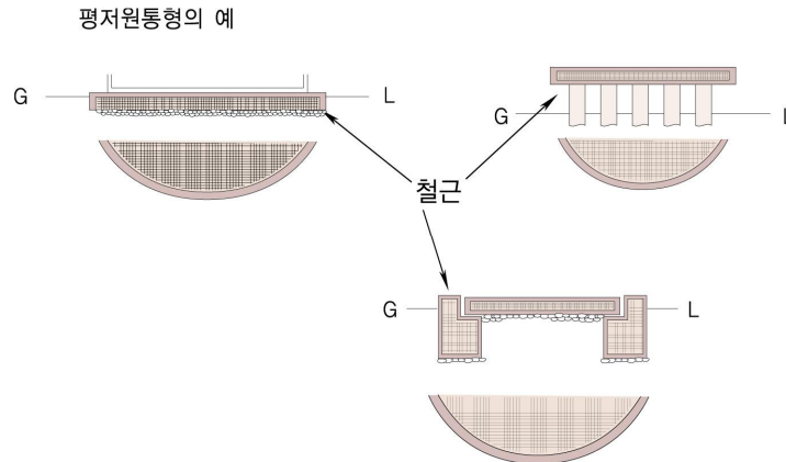
그림 2.2.2.3 저장탱크의 수평기초면
