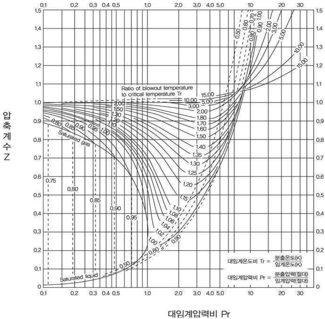
그림 2.6.1.4④ 압축계수
