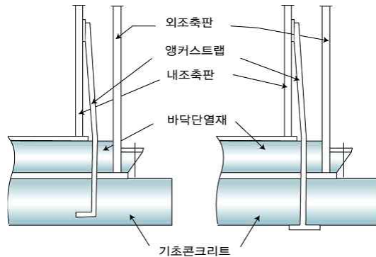
그림 2.2.3.7 평저형 저장탱크의 앵커스트랩 설치방법
