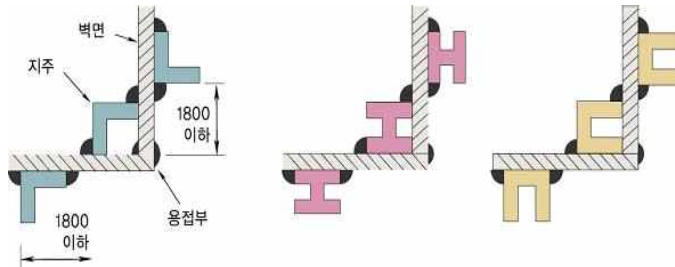
그림 2.7.2.3.4 지주의 설치방법
