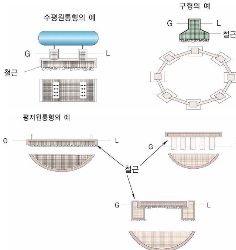
그림 2.2.2.3 저장탱크의 수평기초면
