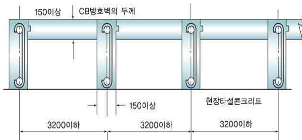
그림 2.7.2.2.2 보조벽의 배치
