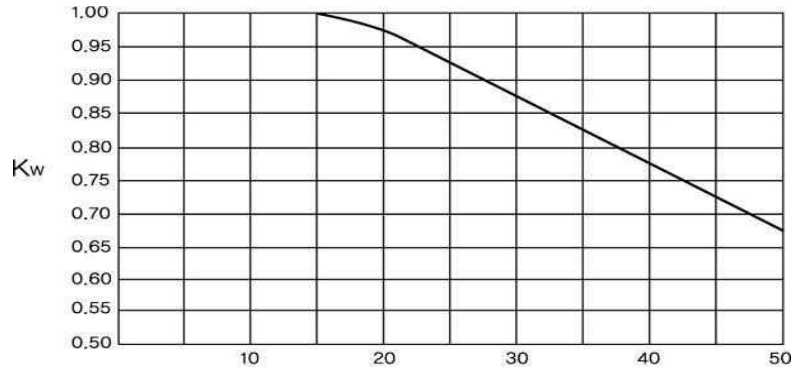
그림 2.6.1.4⑥ 밸런스 벨로우즈형 안전밸브 배압보정계수
