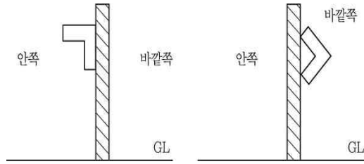
그림 2.7.2.3.2 강관제방호벽의 앵글강 보강
