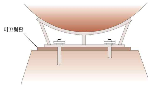
그림 2.2.3.5 미끄럼판의 설치방법
