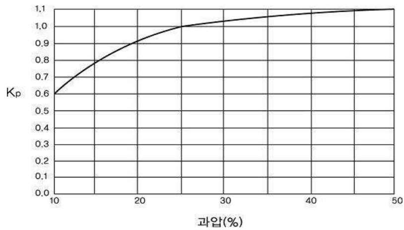
그림 2.6.1.4⑧ 과압보정계수
