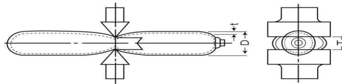
그림 4.4.2.2.1(2)③ 압케시험용 강제썰기
