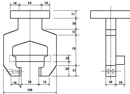
그림 3.11.2.2 밸브 부 착 치 구(예시)
