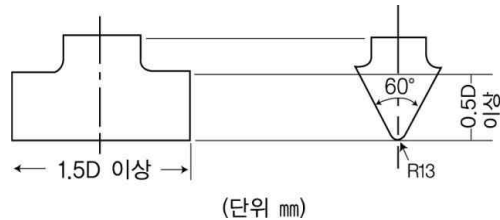
그림 4.4.2.2.1(2)③ 압케시험용 강제썰기
