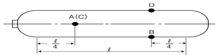
그림 4.4.2.2.1(2)⑤ 두께 측정 방법
