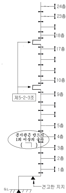
(f) 곡관 2개 설치(24층)
