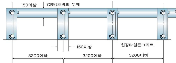
그림 2.9.2.2.2 보조벽의 배치
