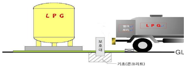
그림 2.3.3.4(6-7) 철근콘크리트 보호대 설치방법 예시
