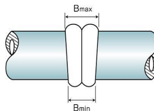
그림 2.5.4.2.2(1)② 융착이음부의 비드폭
