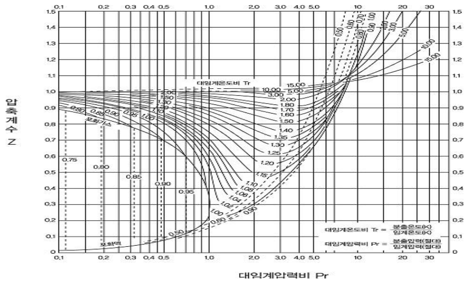
그림 2.8.1.4.1(2)④ 압축계수
