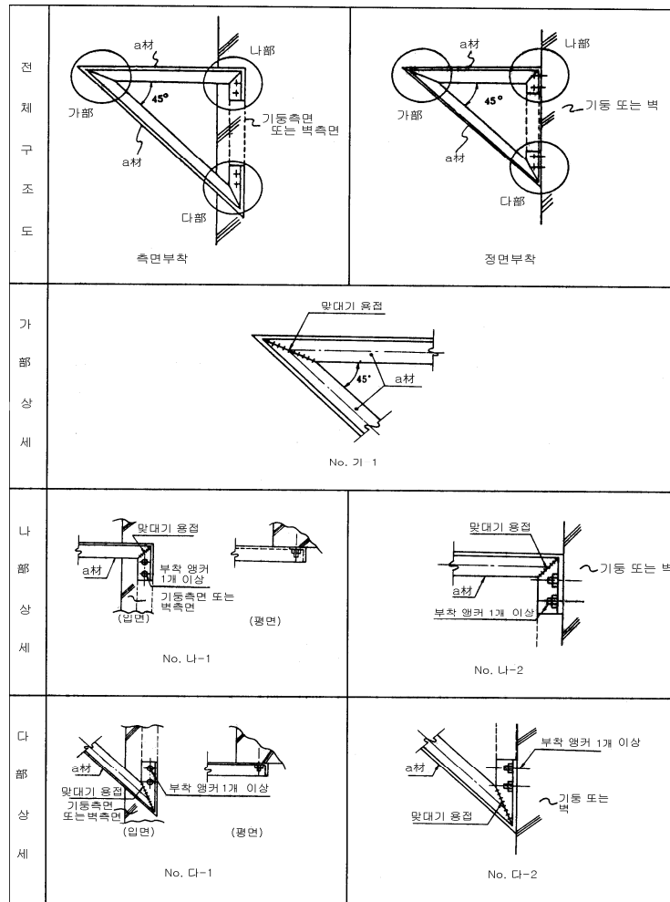
그림 F9.4 횡지관 내진지지구 상세도 및 조립요령
