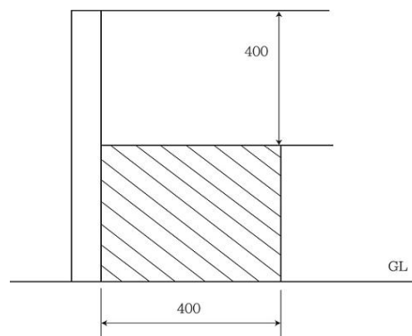
그림 2.9.2.2.3 보조벽의 높이
