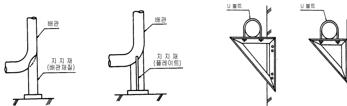
(a) (b) 그림 F8.2 입상관 하부 견고한 지지의 예(자중 및 내진지지 겸용)
