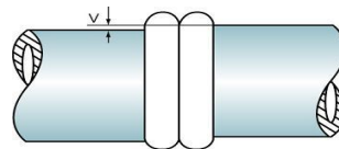
그림 2.5.4.2.2(1)① 융착이음부의 연결오차
