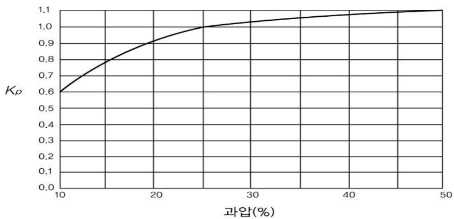
그림 2.8.1.4.1(2)⑧ 과압보정계수
