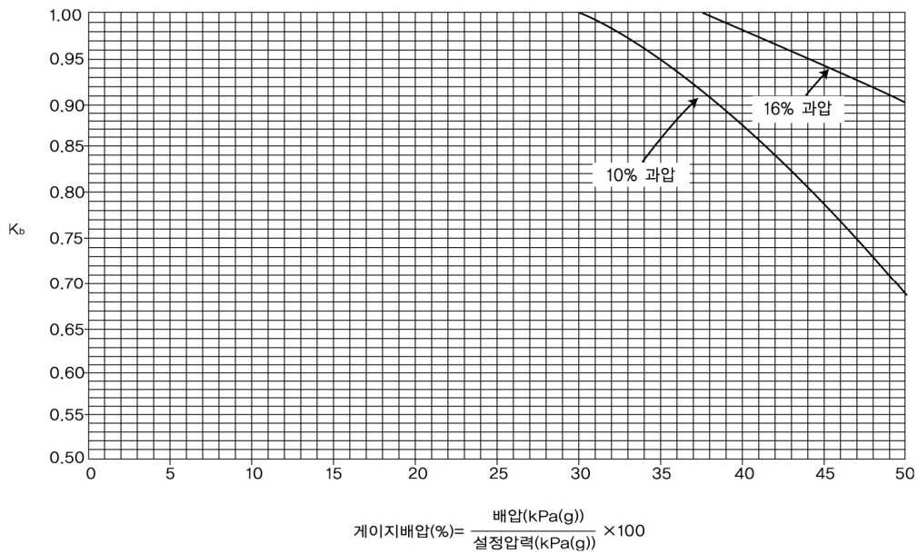
그림 2.6.1.4② 밸런스 벨로우즈형 안전밸브 배압보정계
