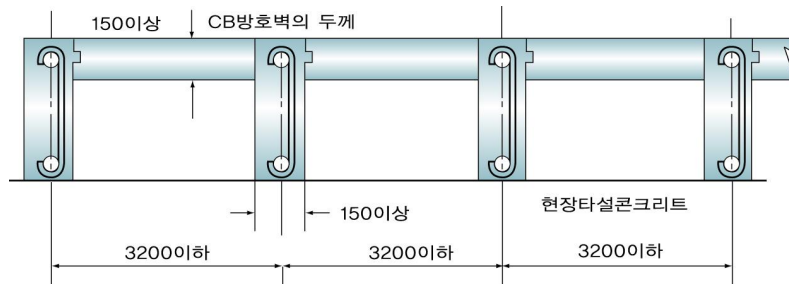
그림 2.7.2.2.2 보조벽의 배치
