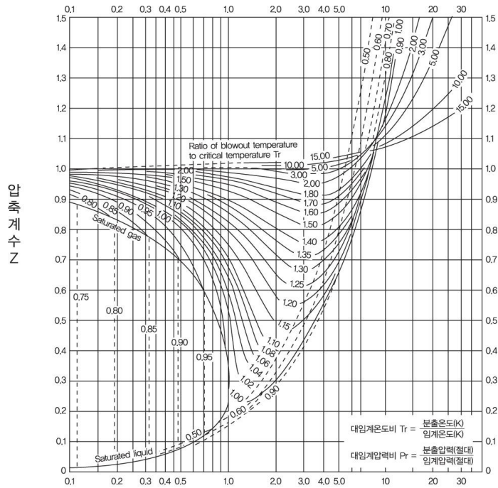
그림 2.6.1.4④ 압축계수
