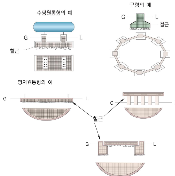
그림 2.2.2.3 저장탱크의 수평기초면
