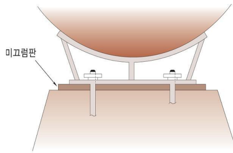
그림 2.2.3.5 미끄럼판의 설치방법
