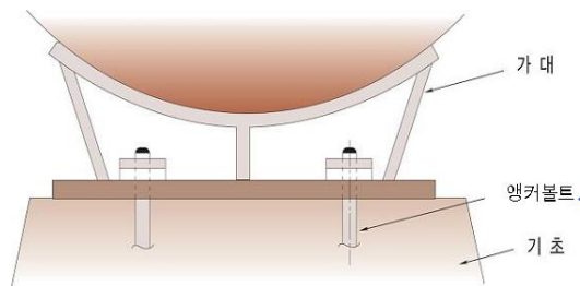
그림 2.2.3.4 앵커볼트의 고정방법
