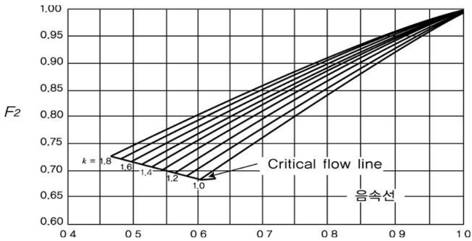
그림 2.8.1.4.1(2)⑤ 이음속계수
