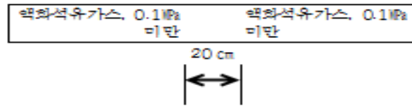
그림 2.5.10.3.1(1) 보호포의 표시방법의 보기
