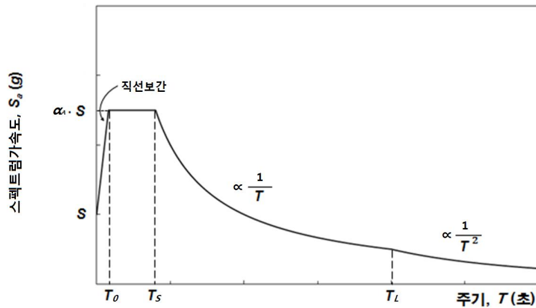
그림 2.4.6.1.1(1) 가속도 표준설계응답스펙트럼(압반지반)
