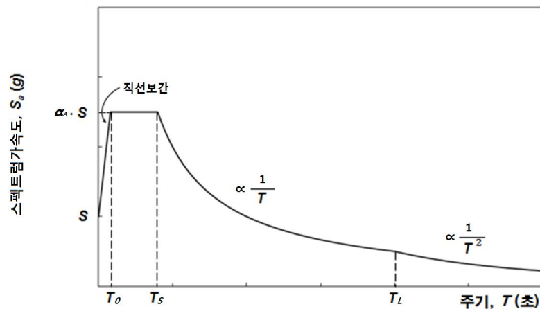
그림 2.4.6.1.1(1) 가속도 표준설계응답스펙트럼(압반지반)
