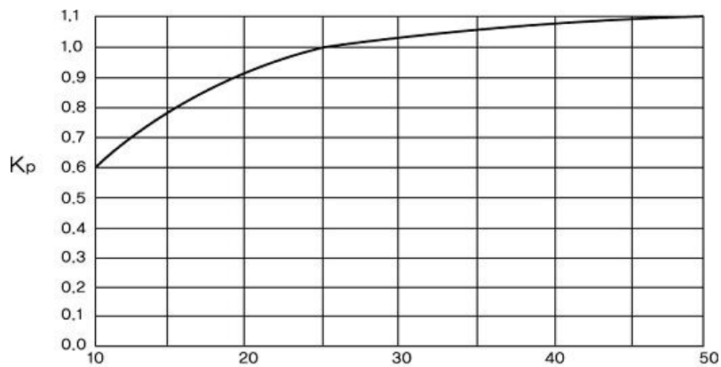
그림 2.6.1.4⑧ 과압보정계수
