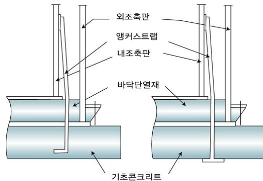
그림 2.2.3.7 평저형 저장탱크의 앵커스트립 설치방법
