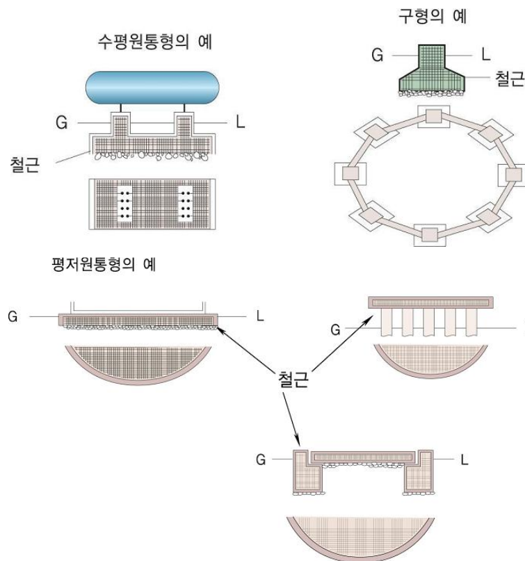
그림 2.2.2.3 저장탱크의 수평기초면
