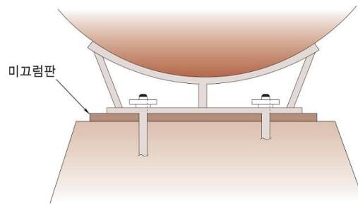
그림 2.2.3.5 미끄럼판의 설치방법
