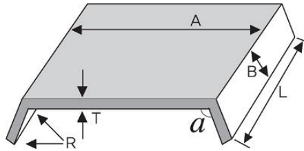
그림 2.5.7.2.3(4) 보호판의 치수 측정
