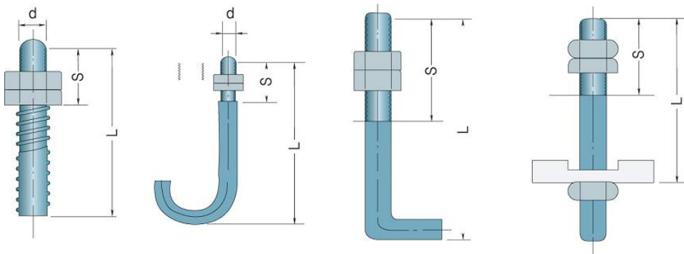
그림 2.2.3.3 앵커볼트의 치수표시 <개정 16.12.15>
