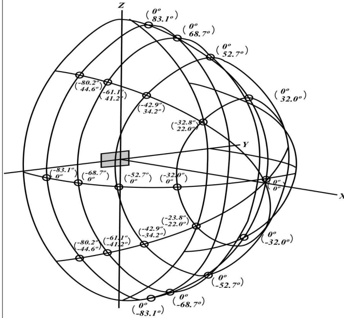
그림 C6 . 방사각도의 측정
