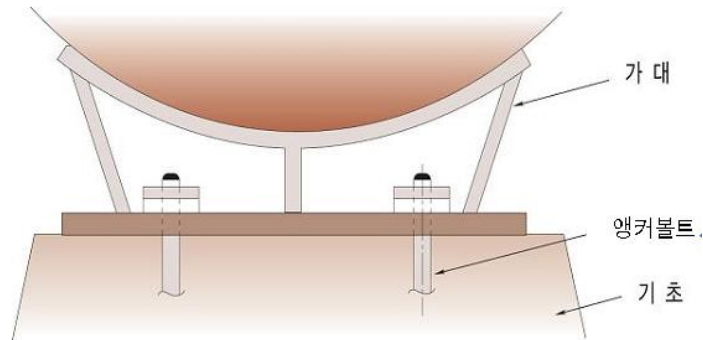
그림 2.2.3.4 앵커볼트의 고정방법
