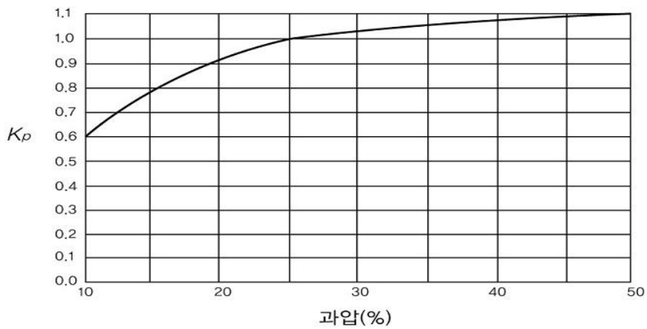
그림 2.8.1.4.1(2)⑧ 과압보정계수
