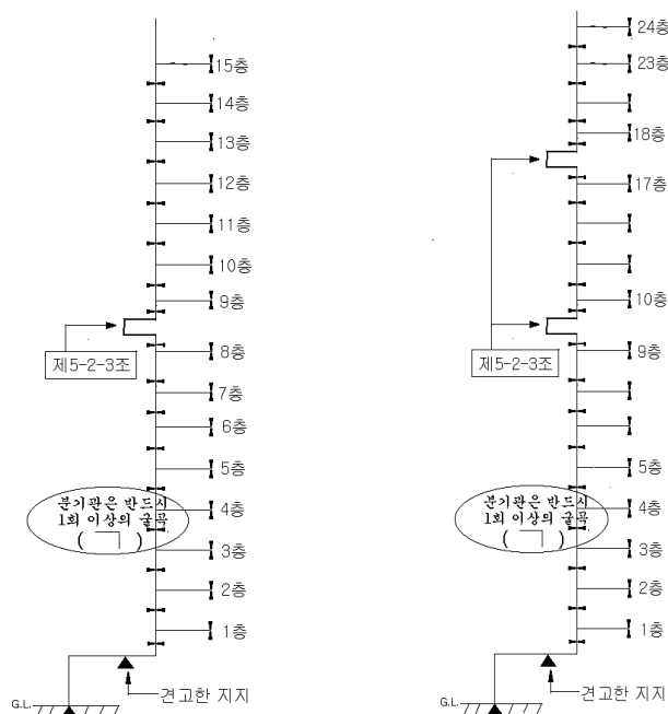
(a) 곡관 1개 설치(15층)
