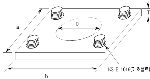
그림 2.3.34(6-3-2) 강판제 보호대의 반침대 설치 방법
