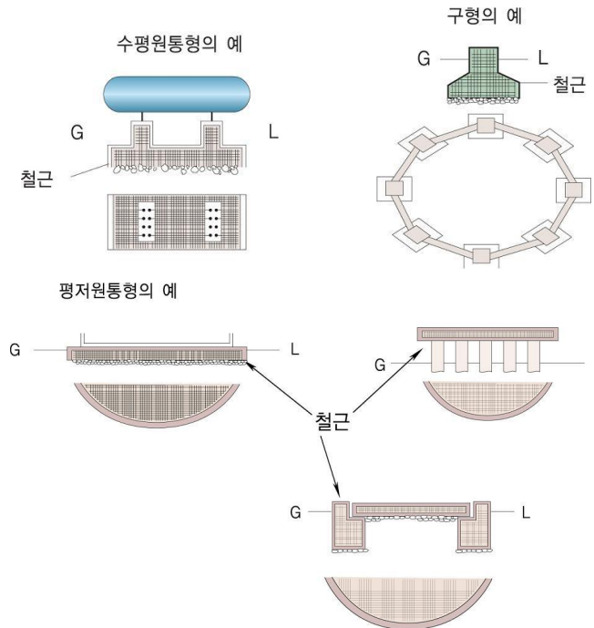
그림 2.2.2.4 저장탱크의 수평기초면
