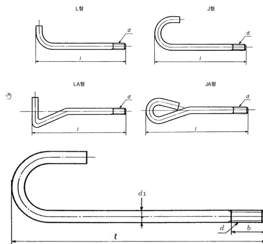
그림 2.2.3.3.1 앵커볼트의 모양
