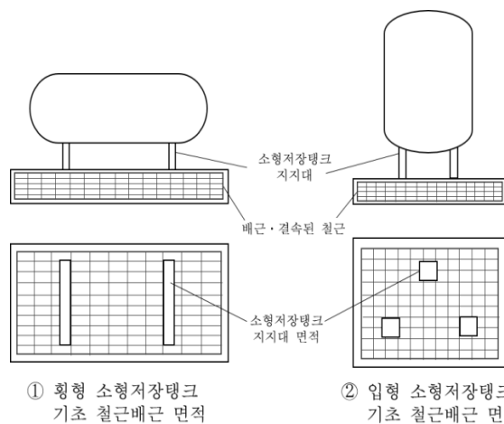
그림 2.3.3.2.3(3-3) 소형저장탱크 일체형 철근콘크리트 기초의 철근배근 예시
