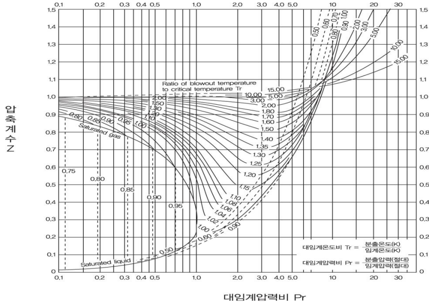
그림 2.8.1.4.1③ Conventional 안전밸브 배압조정계수
