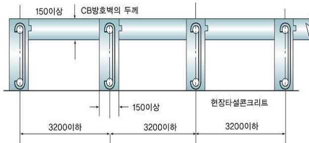
그림 2.9.2.2.2 보조벽의 배치
