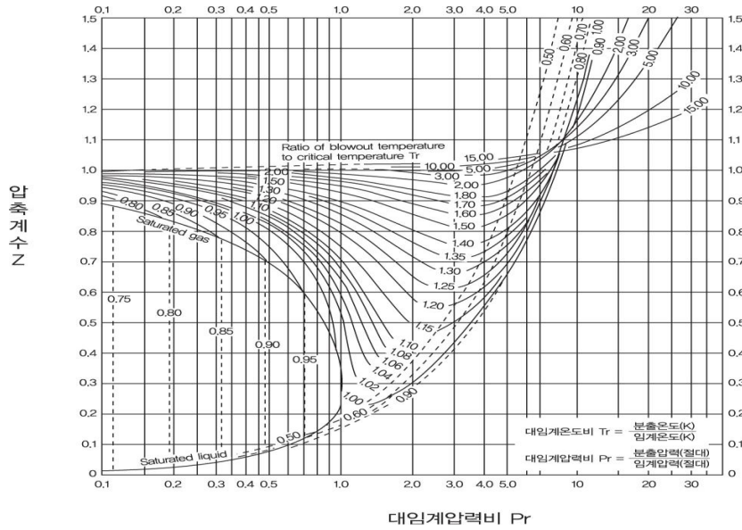
그림 2.8.1.4.1④ 압축계수
