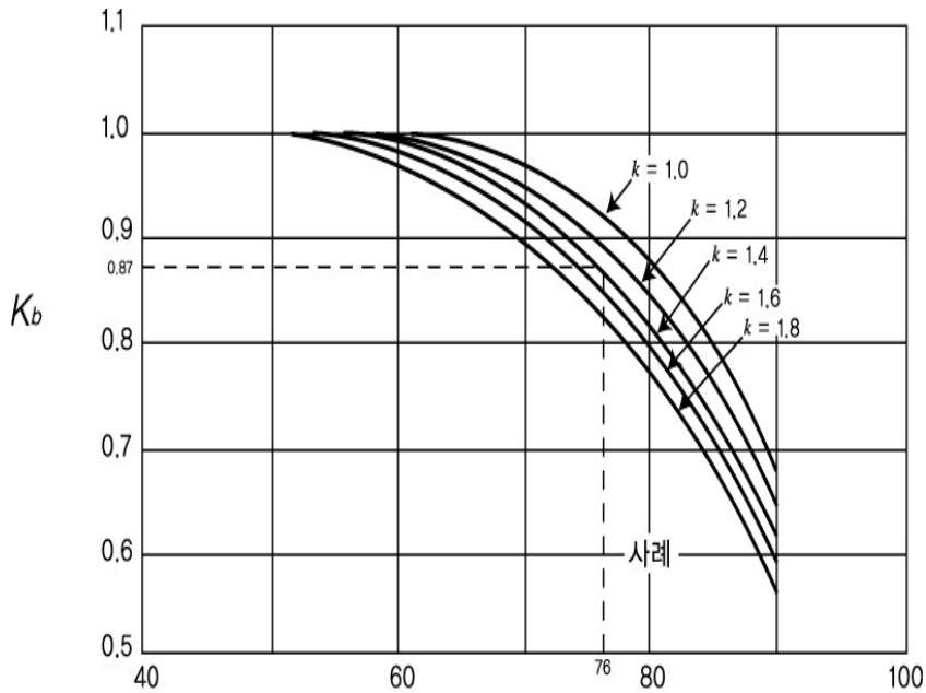
그림 2.8.1.4.1② 벨런스 벨로우즈형 안전밸브 배압보정계수
