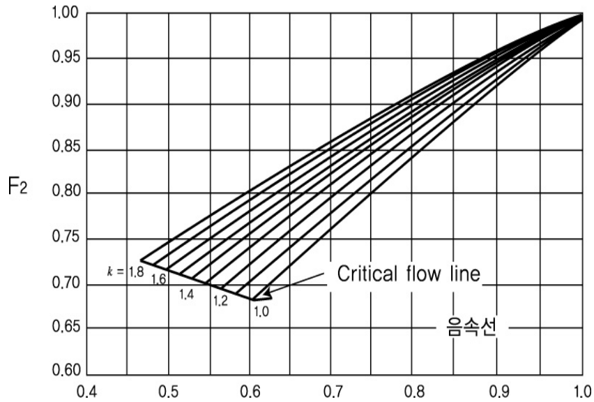
그림 2.8.1.4.1④ 압축계수
