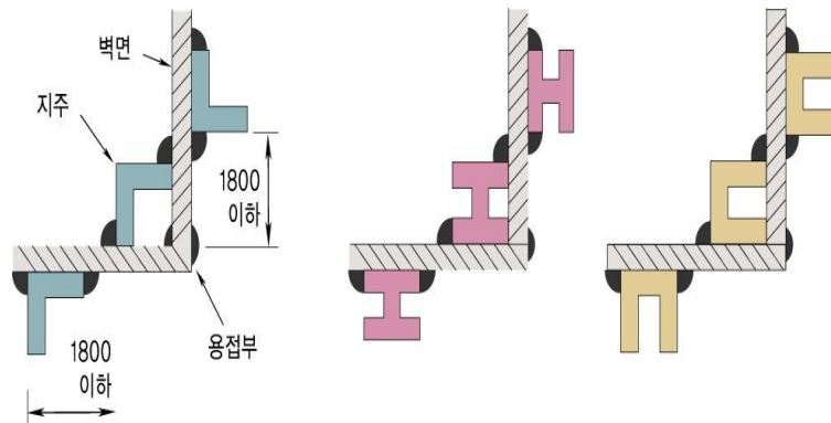
그림 2.9.2.3.4 지주의 설치방법
