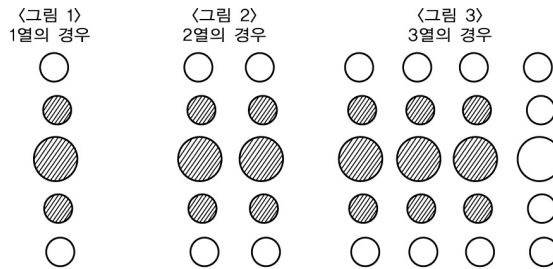
그림 2.9.9.1.4 온도상승방지설비 능력산정기준
