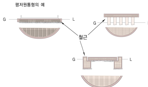
그림 2.2.2.3 저장탱크의 수평기초면
