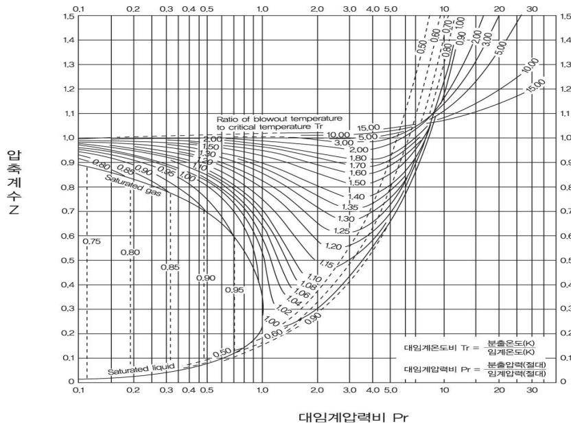
그림 2.8.1.4.1④ 압축계수
