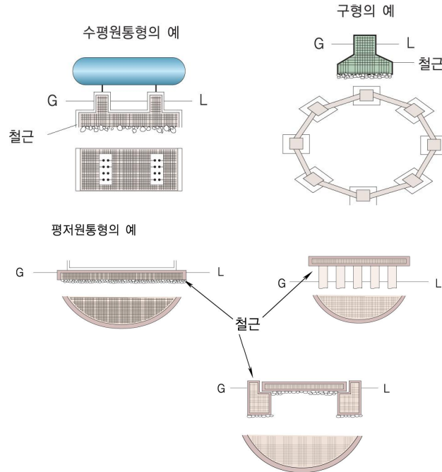
그림 2.2.2.3 저장탱크의 수평기초면
