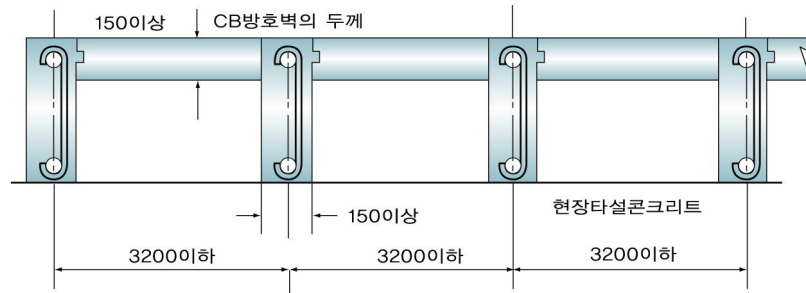
그림 2.8.2.2.2 보조벽의 배치
