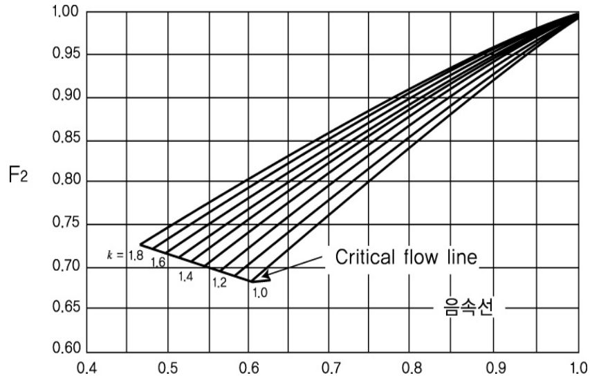
2.7.1.4.1⑤ 아음속계수
