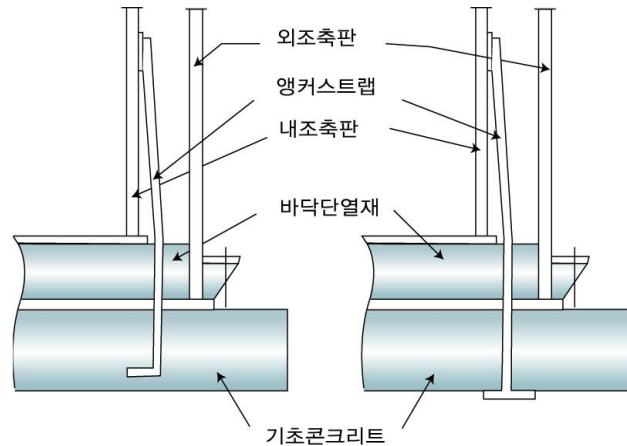
그림 2.2.3.7 평저형 저장탱크의 앵커스트랩 설치방법
