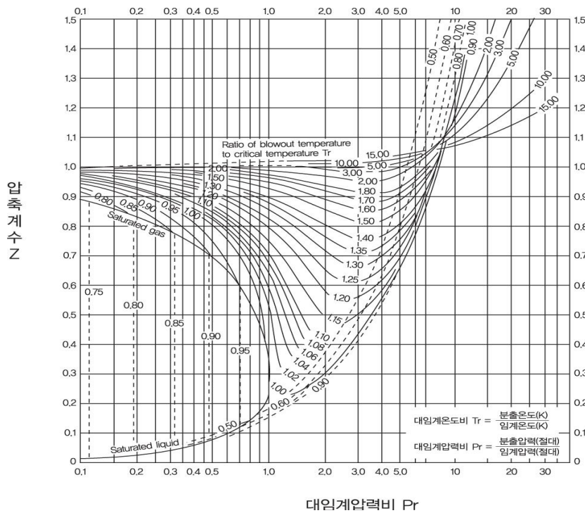
그림 2.7.1.4.1④ 압축계수
