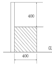
그림 2.8.2.2.3 보조벽의 높이
