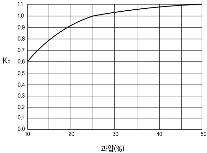
그림 2.7.1.4.2③ 과압보정계수
