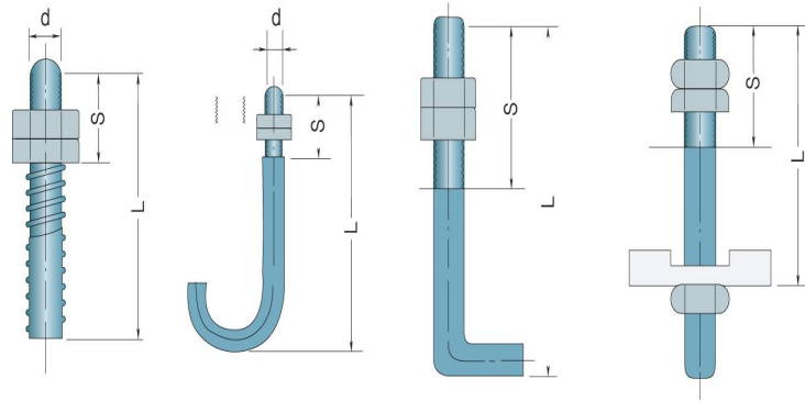
그림 2.2.3.3 앵커볼트의 치수표시 <개정 17.8.7>
