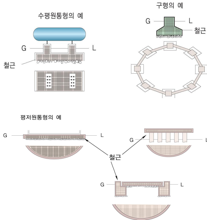
그림 2.2.2.3 저장탱크의 수평기초면
