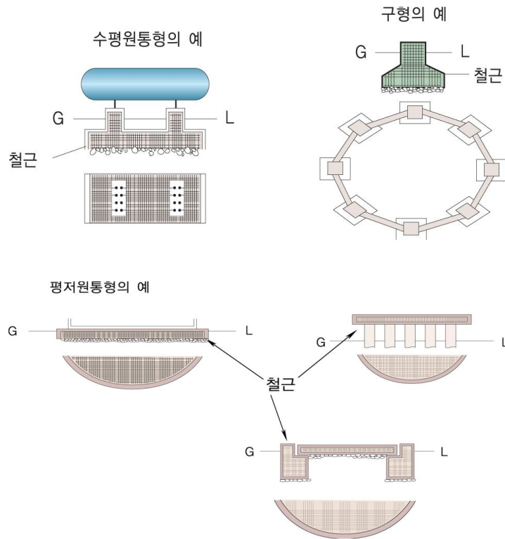
그림 2.2.2.3 저장탱크의 수평기초면
