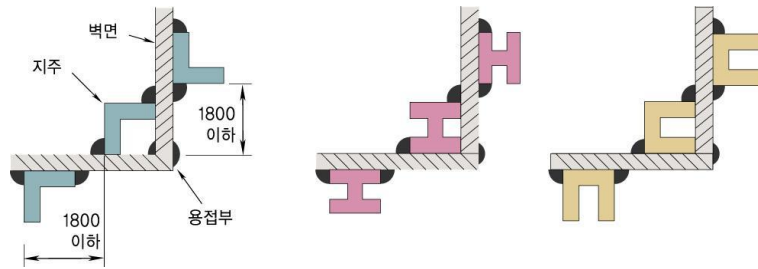
그림 2.7.2.3.4 지주의 설치방법
