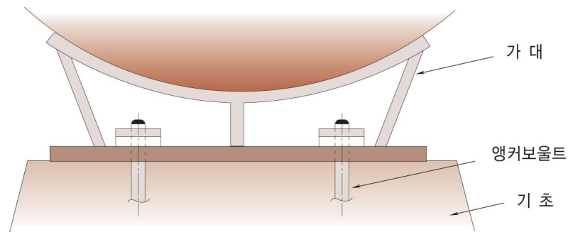
그림 2.2.3.4 앵커보울트의 고정방법
