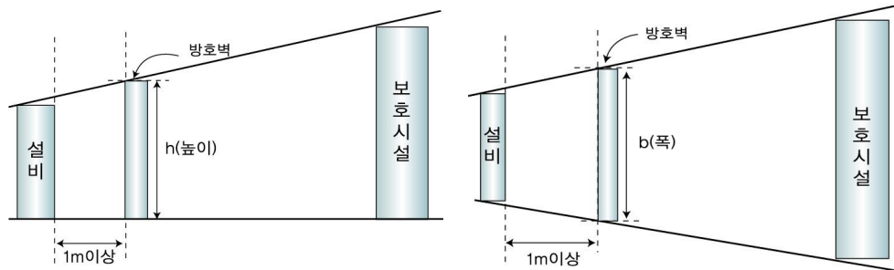
그림 2.7.2.1.1① 방호벽 설치 예(측면도)
