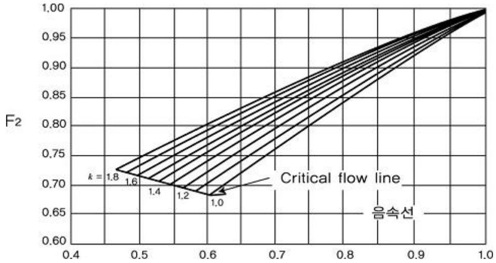
그림 2.6.1.4⑤ 아음속계수
