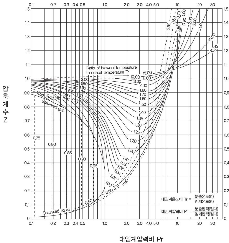
그림 2.6.1.4④ 압축계수
