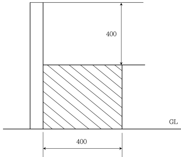
그림 2.7.2.2.3 보조벽의 높이
