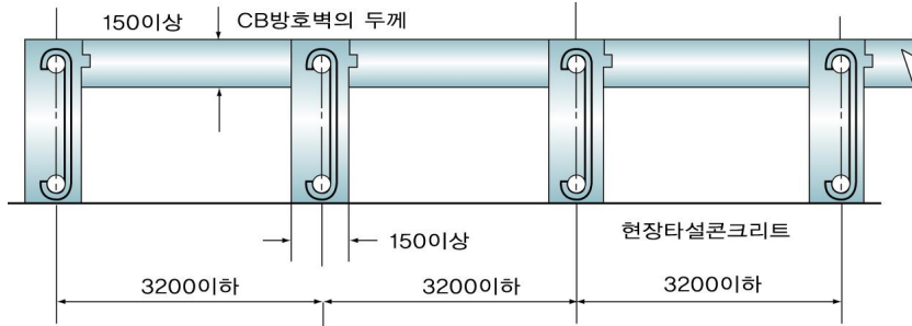
그림 2.7.2.2.2 보조벽의 배치
