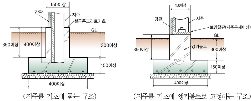
그림 2.7.2.3.6 강관제 방호벽의 고정방법 보기
