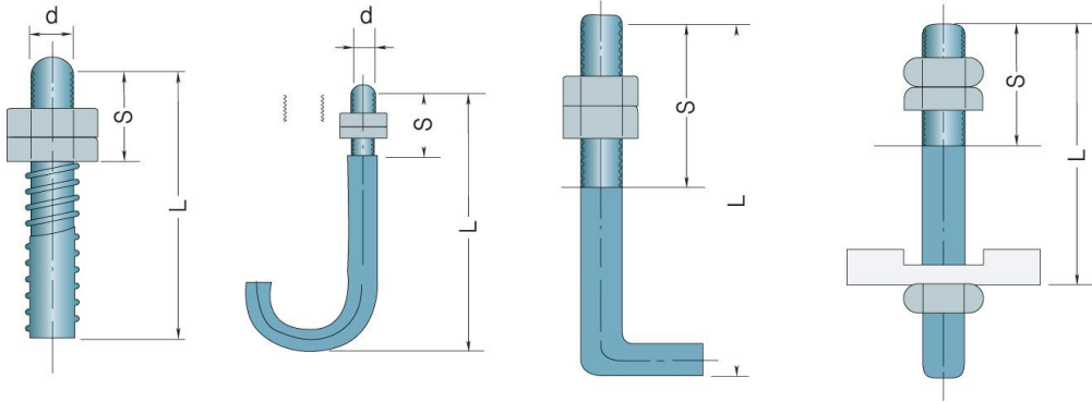
그림 2.2.3.3 앵커보울트의 치수표시
