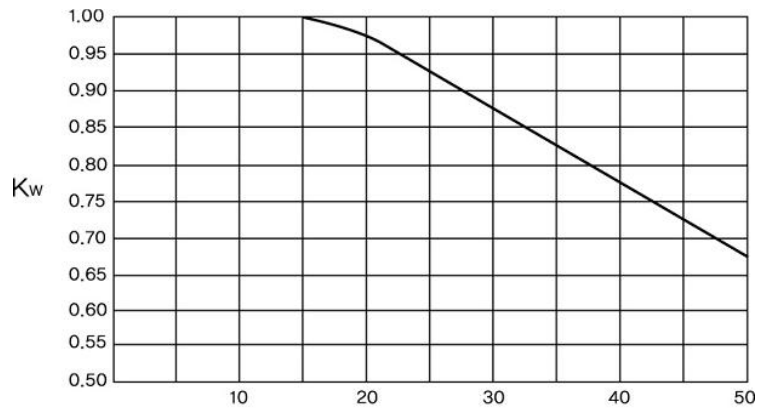
그림 2.6.1.4⑤ 아음속계수
