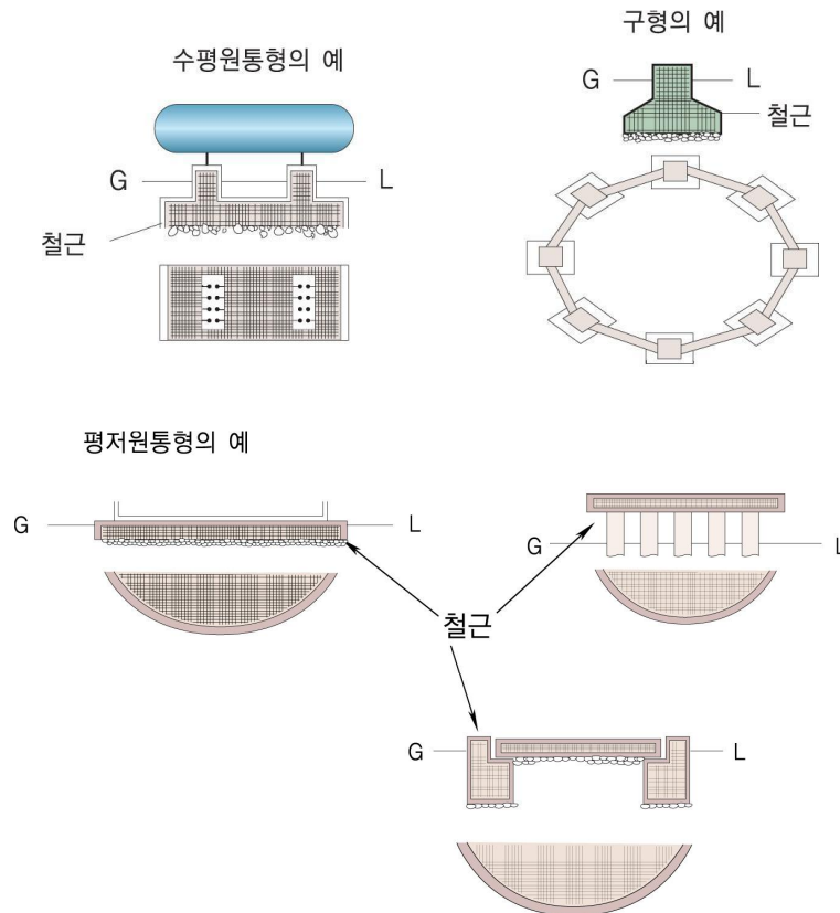
그림 2.2.2.3 저장탱크의 수평기초면
