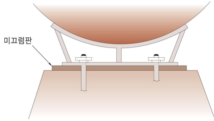
그림 2.2.3.5.3 미끄럼판의 설치방법
