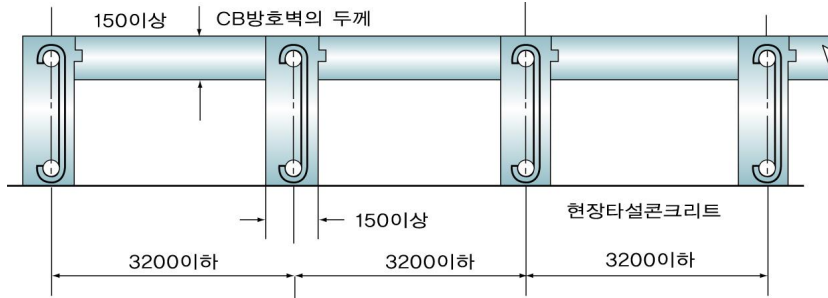
그림 2.7.2.2.2 보조벽의 배치
