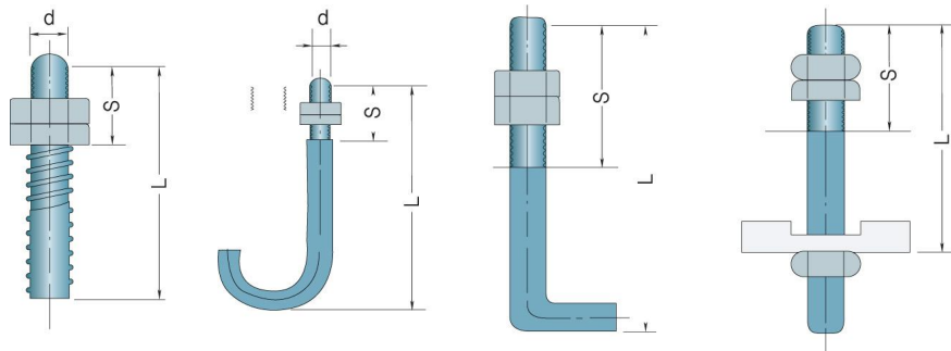
그림 2.2.3.3 앵커보울트의 치수표시
