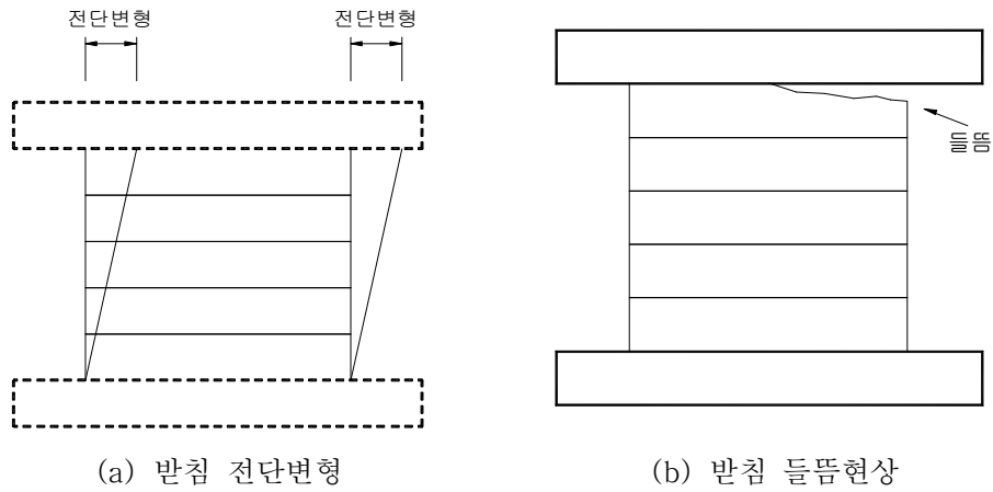
그림 A7.2.6 받침 전단변형 및 들뜸현상 예
