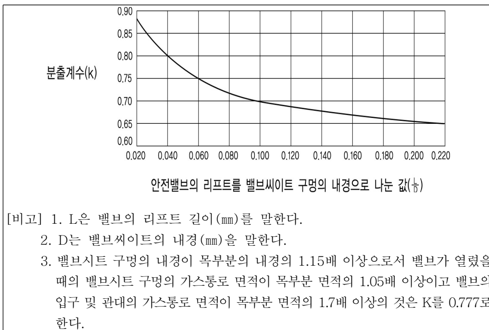
그림 2.6.1.1.4 분출계수
