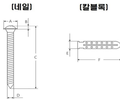
그림 2.5.10.3.2(5-3) 네일형 라인마크의 모양·크기 및 표시방법
