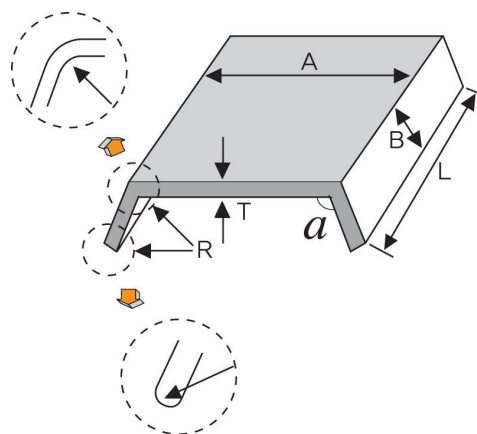
그림 2.5.7.2.7 보호판의 치수
