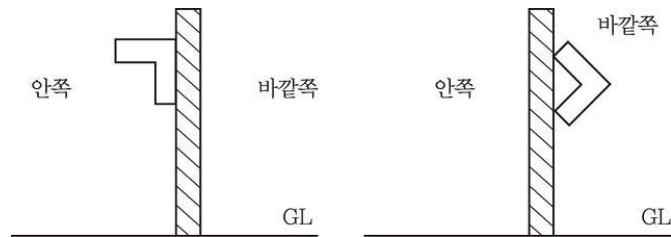
그림 2.7.2.3.2 강판제한방호벽의 앵글강 보강
