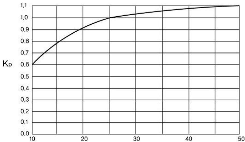
그림 2.6.1.4⑧ 과압보정계수
