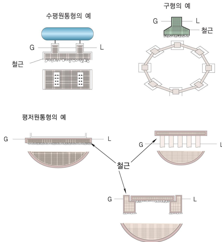
그림 2.2.2.3 저장탱크의 수평기초면
